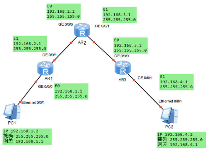
图 3.1-1 实验拓扑图
